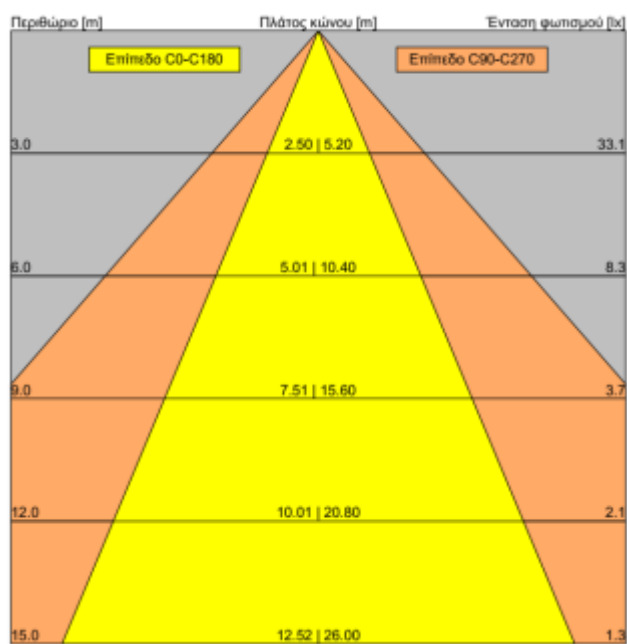
Εικόνα Β.2.12.β Ενδεικτικό διάγραμμα κώνου Φωτεινής Έντασης (φ/σ ενδεικτικού τύπου)
