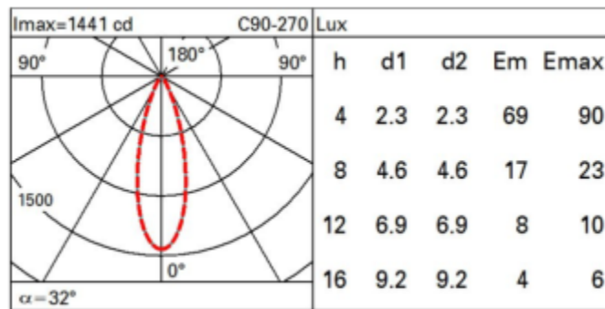
Εικόνα Β.2.1. Ενδεικτικό πολικό διάγραμμα Φωτεινής Έντασης (φ/σ ενδεικτικού τύπου)
