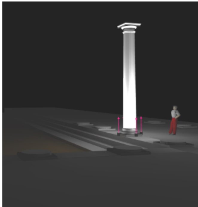
Εικόνα Β.2.18.ε Ενδεικτική 3D Κατανομή λαμπρότητας της θέσης του κίονα του Α διαδρόμου (φ/σ ενδεικτικού τύπου)
