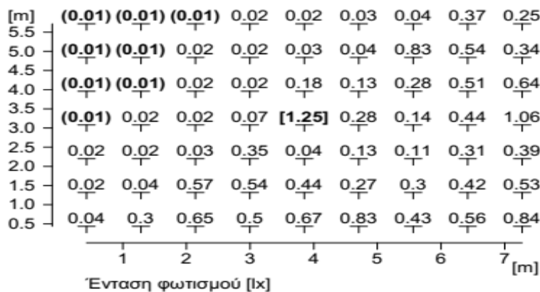
Εικόνα B.2.20.ζ Επισκόπηση αποτελεσμάτων έντασης φωτισμού σε πίνακα (δάπεδο πλατείας ΝΑ γωνία κρηπίδας)
