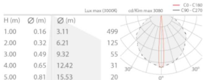
Εικόνα Β.2.20.α Ενδεικτικό πολικό διάγραμμα Φωτεινής Έντασης (φ/σ ενδεικτικού τύπου)
