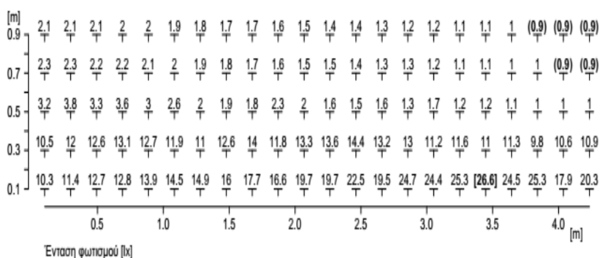
Εικόνα B.2.20.στ Επισκόπηση αποτελεσμάτων έντασης φωτισμού σε πίνακα (νότια πλευρά κρηπίδας)
