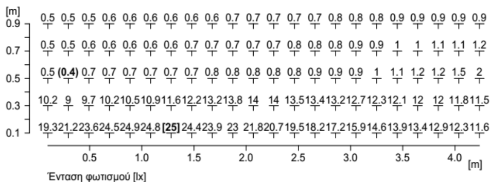
Εικόνα B.2.20.ε Επισκόπηση αποτελεσμάτων έντασης φωτισμού σε πίνακα (ανατολική πλευρά κρηπίδας)
