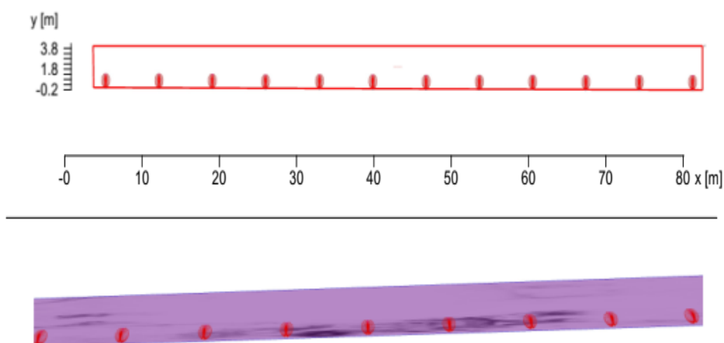
Εικόνα Β.2.25.β Ενδεικτική τοποθέτηση του σημειακών φωτιστικών στη νότια πλευρά του εμπορικού δρόμου
