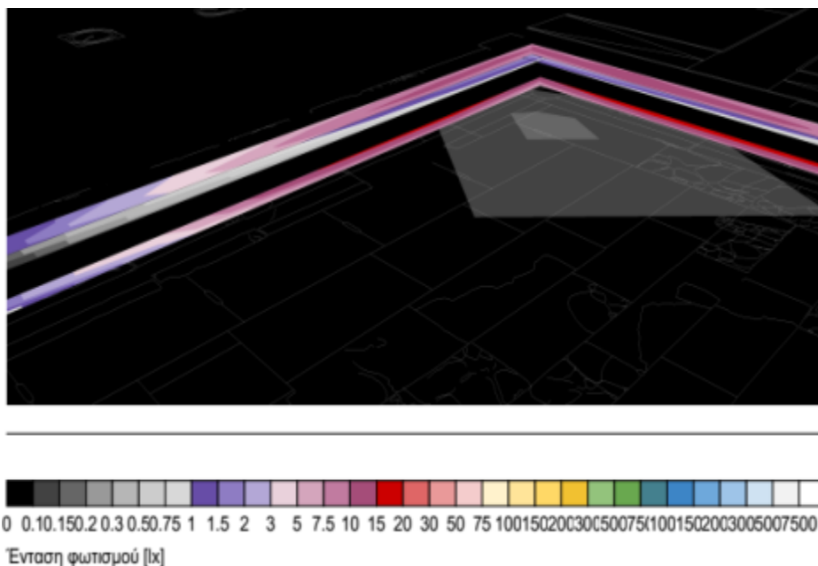
Εικόνα Β.2.20.η Ενδεικτική Κατανομή λαμπρότητας μέσω ψευδοχρωμάτων (φ/σ ενδεικτικού τύπου)
