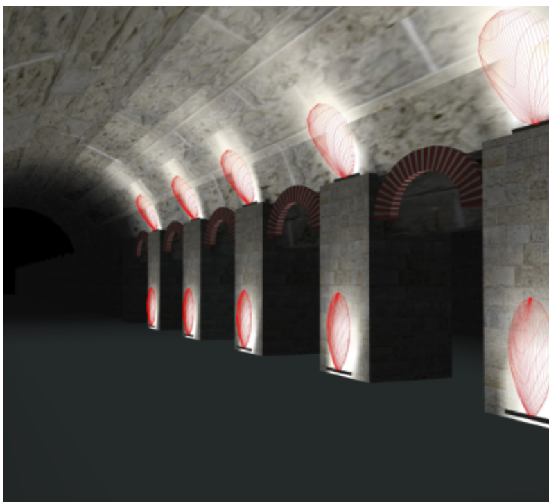
Εικόνα Β.2.12.στ Ενδεικτική 3Δ Κατανομή λαμπρότητας σε πεσσούς και οροφή θόρειας στοάς (φ/σ ενδεικτικού τύπου)
